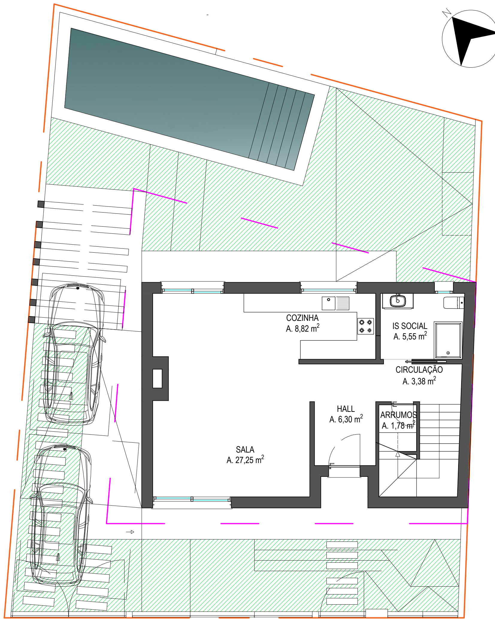
PLANTA PISO 0
